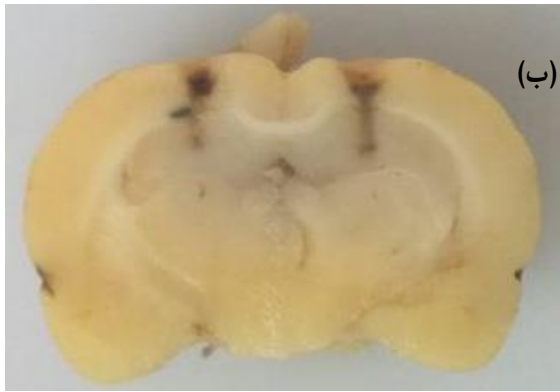
شکل ۱- برش کروئال مغز موش بزرگ آزمایشگاهی در موقعیت ۳/۸۴- از برگما (الف) تصویر شماتیک برش کروئال بر اساس اطلس پاکسینوس و واتسون (ب) نمونه برش کروئال مغز موش بزرگ آزمایشگاهی در موقعیت شکنج دندانهای.
