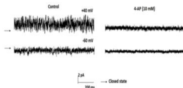
شکل ۳- اثر 4-AP بر فعالیت تک کانال حساس به 4-AP در ولتاژهای +4 mV و -60 mV. ثبت از فعالیت کانال در +40 mV (در شرایط 50 mM کلریدپتاسیم در فضای ترانس و 200 mM کلریدپتاسیم در فضای سیس) قبل و بعد از اضافه کردن 4-آمینوپیریدین با غلظت 10 mM به فضای سیس. 4-آمینوپیریدین به طور کامل فعالیت کانال را مهار می‌کند (n = 3).
