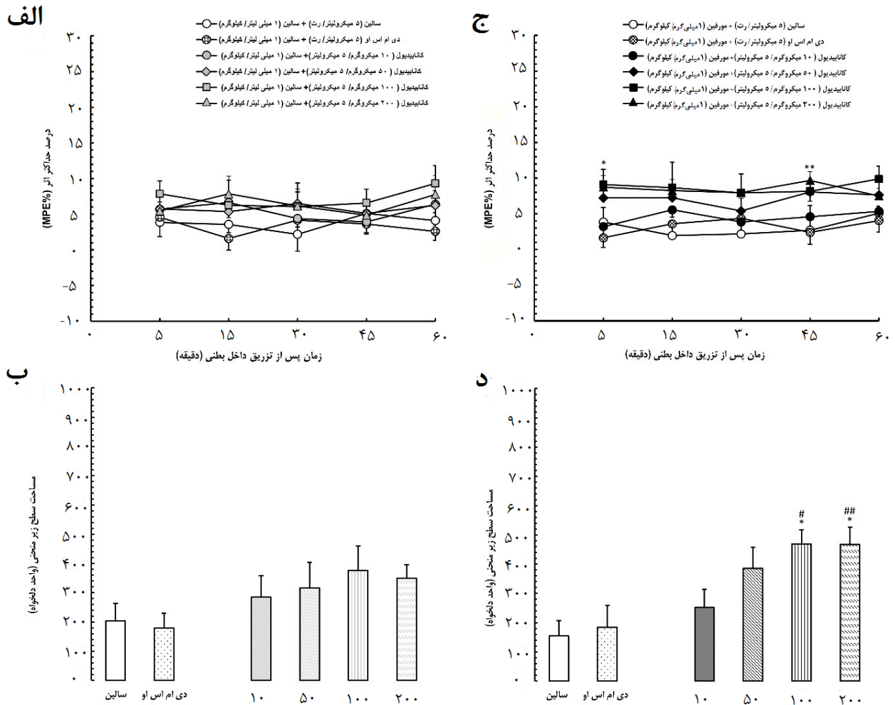
شکل ۳- اثر کانابیدیول بر پاسخ ضددردی در غیاب استرس و در حضور مورفین. (الف): درصد حداکثر اثر در گروه‌های دریافت‌کننده سالیین، DMSO و کانابیدیول (۱۰، ۵۰، ۱۰۰ و ۲۰۰ میکروگرم) در غیاب استرس تفاوت معنی‌داری نشان نداد. (ب): تحلیل مساحت سطح زیر منحنی نیز عدم تفاوت معنی‌دار بین گروه‌ها را تأیید کرد. (ج): در حضور مورفین (۱ میلی‌گرم/کیلوگرم)، تجویز کانابیدیول موجب افزایش وابسته به دوز پاسخ ضددردی شد، به‌طوری‌که دوزهای ۱۰۰ و ۲۰۰ میکروگرم افزایش معنی‌داری نسبت به گروه DMSO نشان دادند. (د): تحلیل مساحت سطح زیر منحنی نیز افزایش معنی‌دار پاسخ در دوزهای بالاتر کانابیدیول را تأیید کرد. هر نقطه نشان‌دهنده میانگین \pm خطای استاندارد میانگین برای ۶-۷ حیوان است. *تفاوت معنی‌دار با گروه DMSO با p < 0.05 ، **تفاوت معنی‌دار با گروه DMSO با p < 0.01 ، ##تفاوت معنی‌دار با گروه سالیین با p < 0.05 ، ###تفاوت معنی‌دار با گروه سالیین با p < 0.01 .
