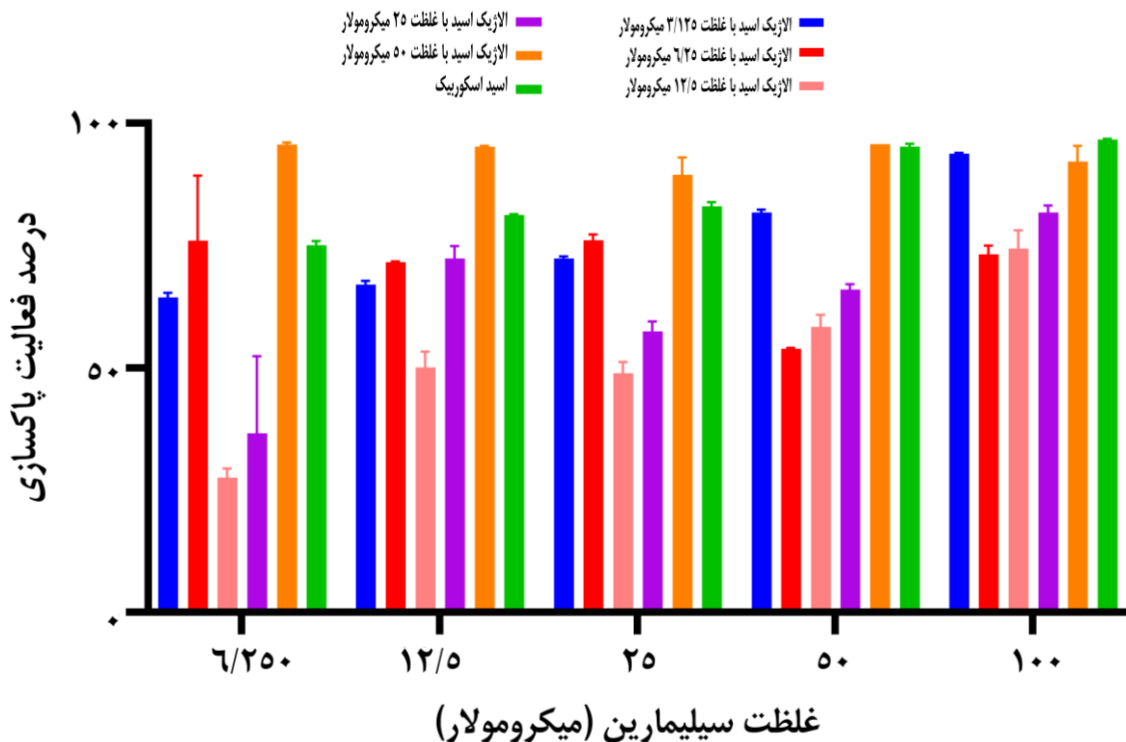
نمودار ۴- فعالیت پاکسازی رادیکال آزاد DPPH توسط ترکیب همزمان غلظت‌های مختلف سیلیمارین و الایژیک‌اسید در مقایسه با اسیداسکوربیک به‌عنوان نمونه استاندارد. سه آزمایش مستقل در سه تکرار انجام شد و داده‌ها به‌صورت میانگین \pm SD نشان داده شده است.
